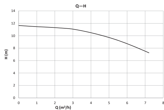
Basic 25-12Z
